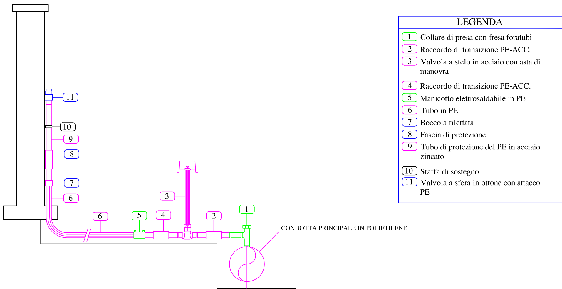
PARTICOLARE ATTACCO GAS (1:20)
